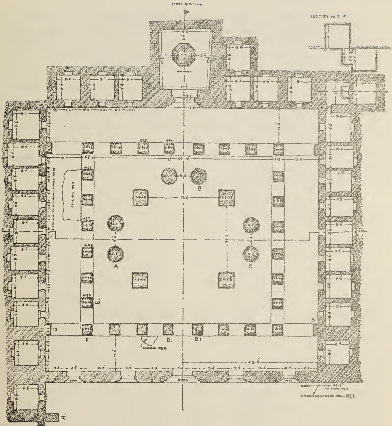
Fig. 6. Bāgh, Cave IV: Plan.
