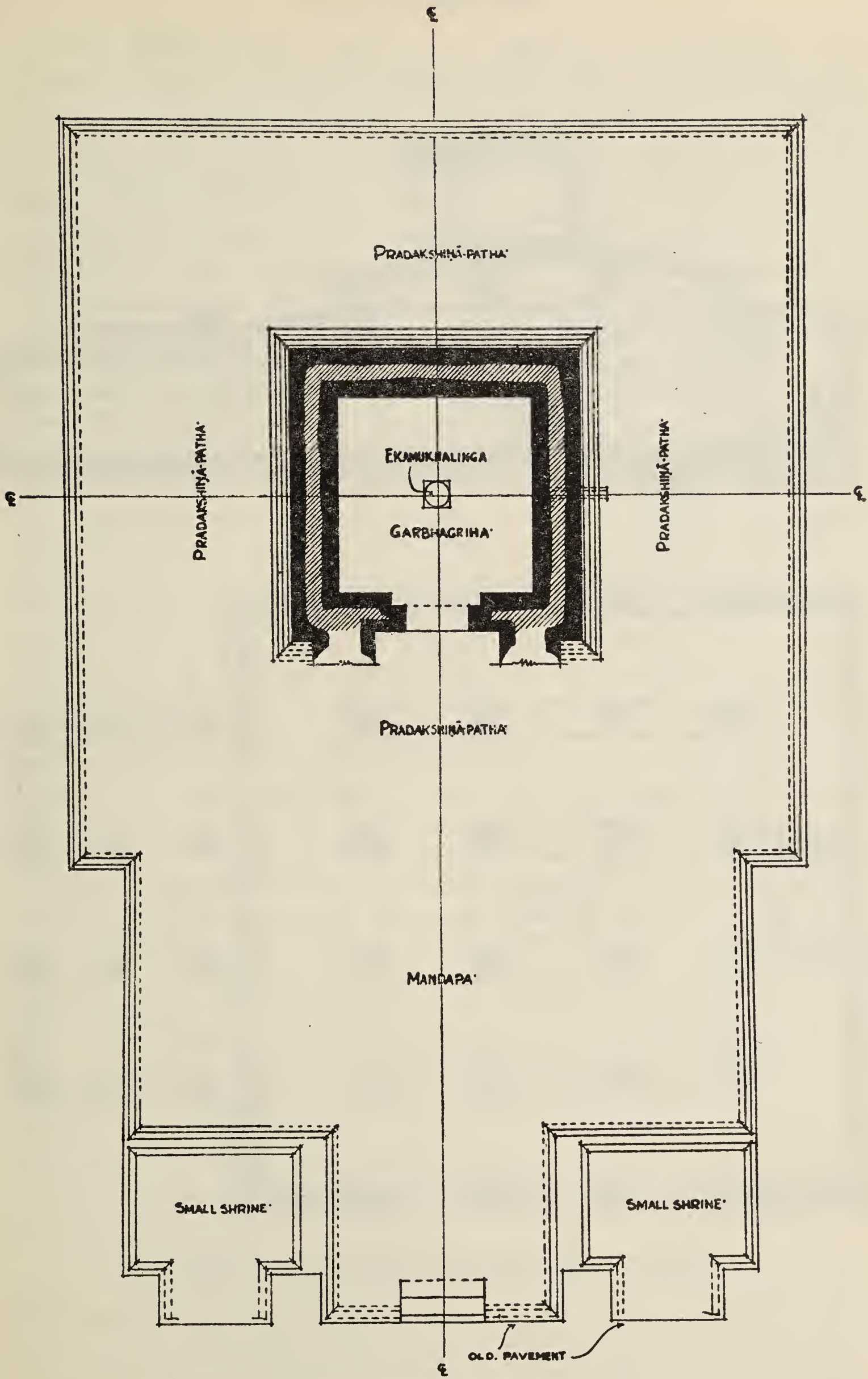
Fig. 23. Bhūmarā, Śiva temple: Plan.
