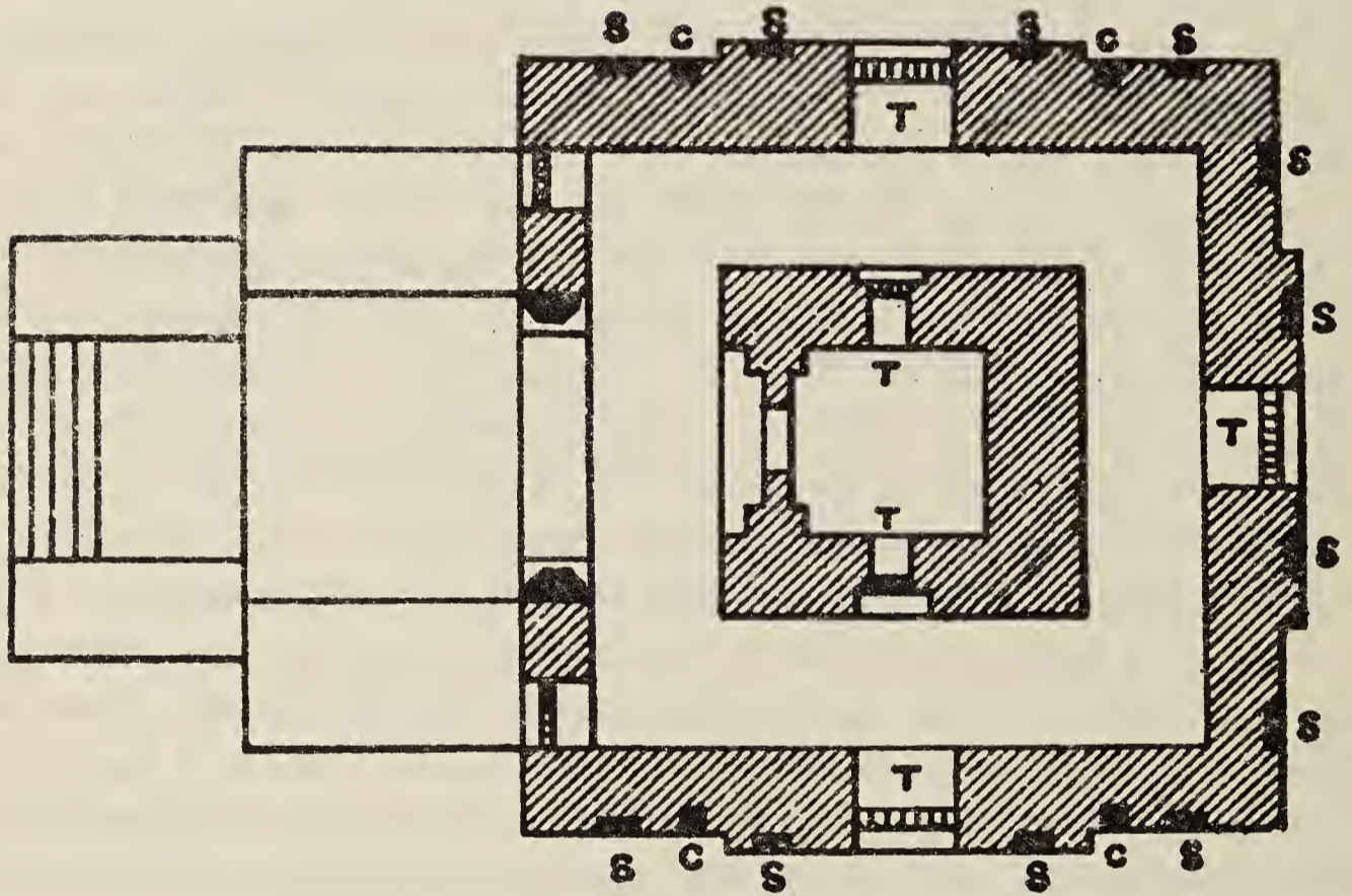
Fig. 22. Nāchnā Kuṭhārā, Pārvati temple: Plan.
