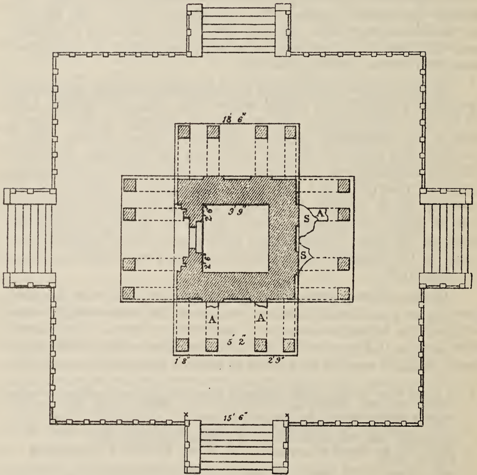
Fig. 25. Deogarh, Daśavatāra temple: Plan.
