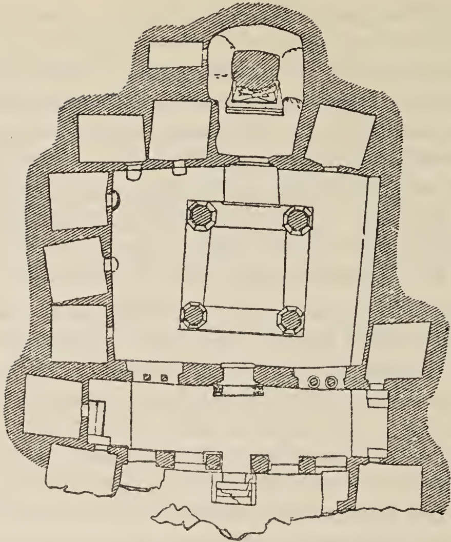
Fig. 1. Ajaṅṭā, Cave XI: Plan.
