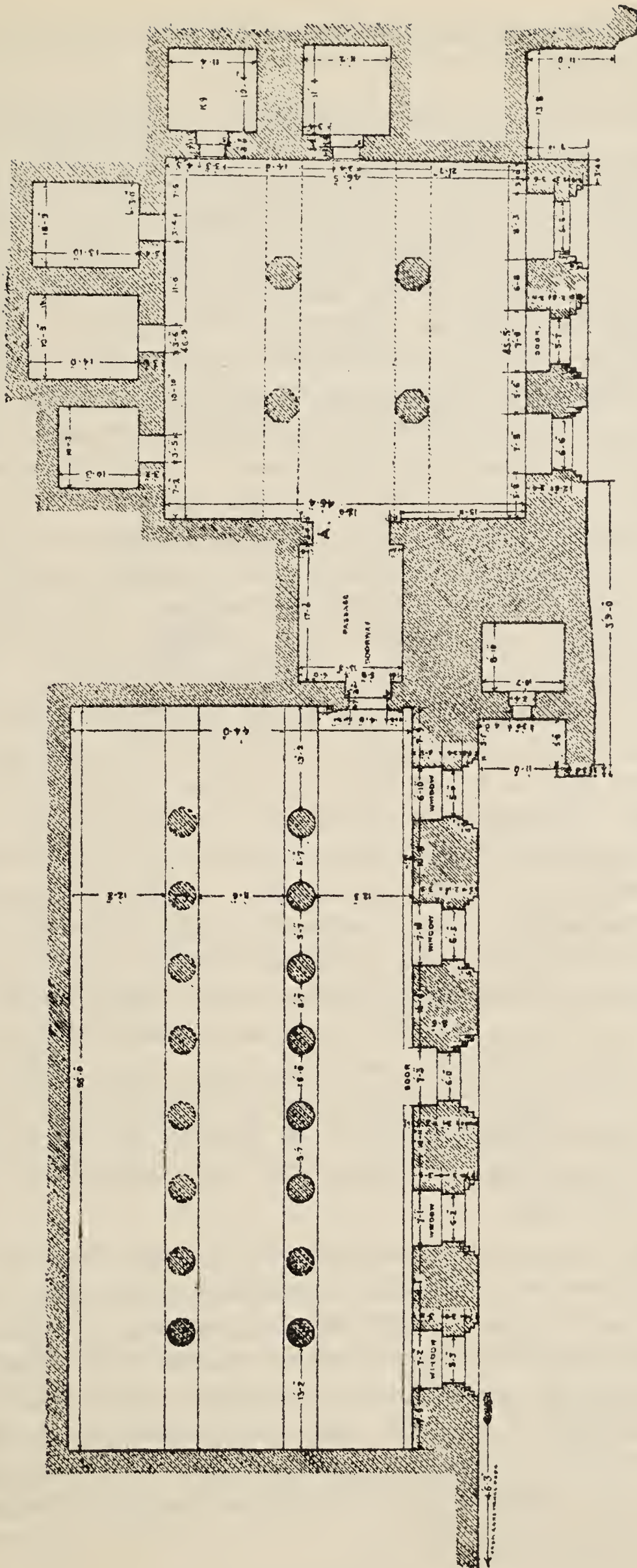
Fig. 7. Bāgh, Caves V & VI: Plan.
